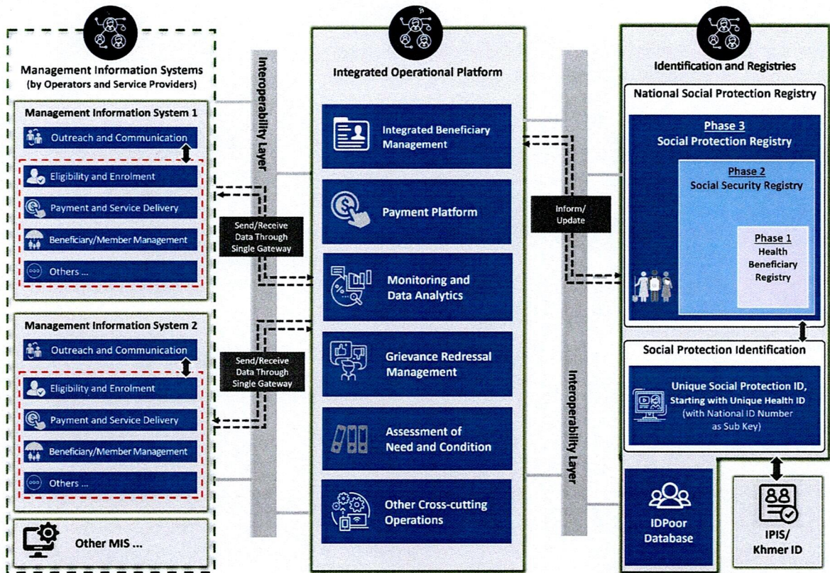
ដ្យាក្រាម៖ និម្មាបនកម្មប្រព័ន្ធ ICT សម្រាប់ប្រព័ន្ធគាំពារសង្គមកម្ពុជា
